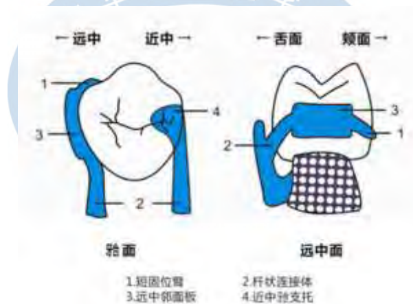
图8 板杆卡环
